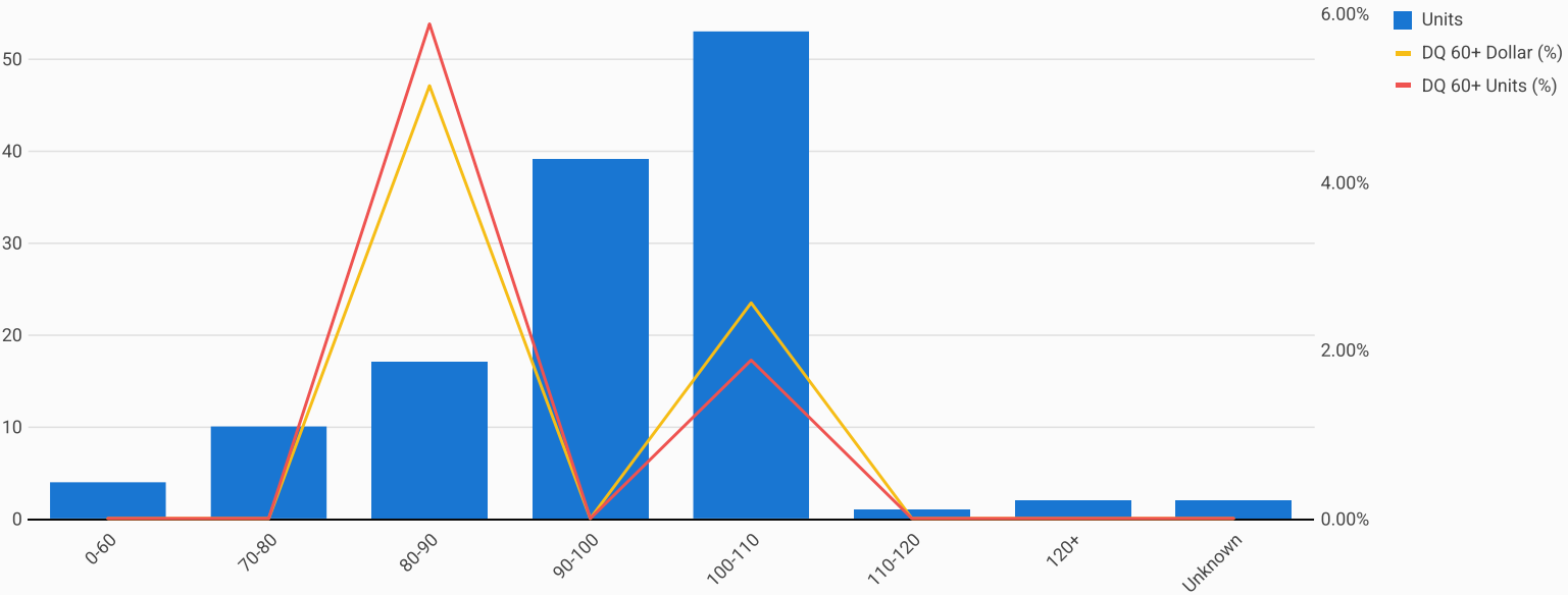
DQ 60+ Percentage by LTC Bucket
